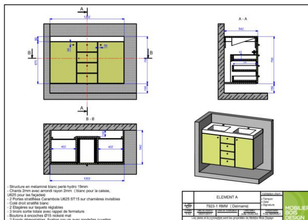
Plan d'exécution
